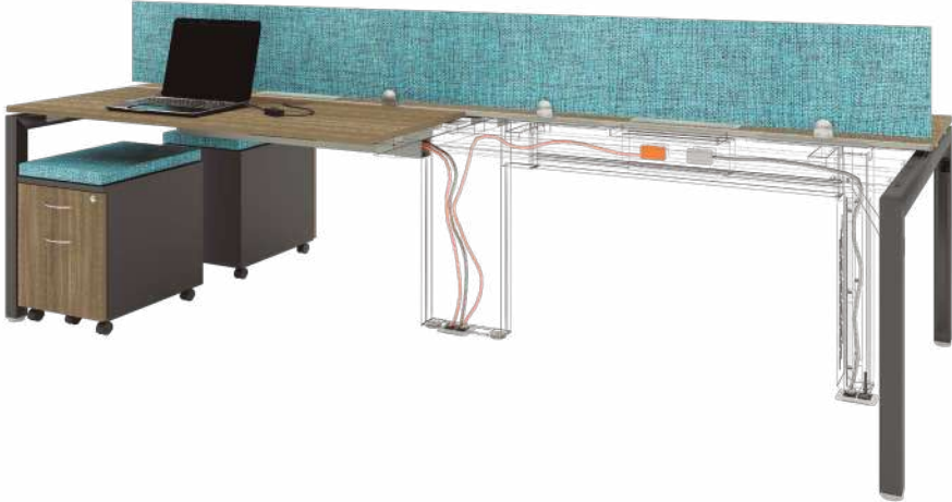
Módulo operativo con conexión convencional a través de soportes y charolas.
